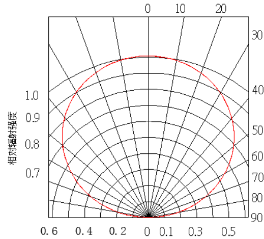
图5: 角度和辐射强度
